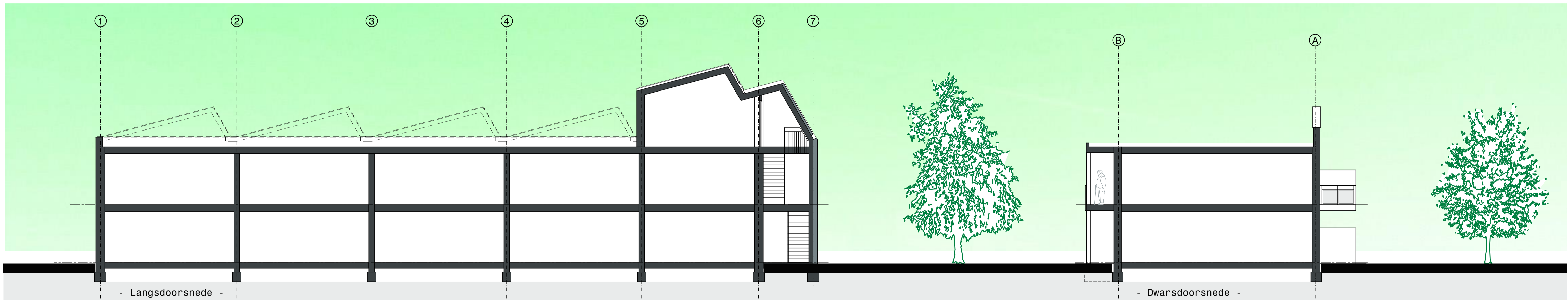
- Langsdoorsnede -
