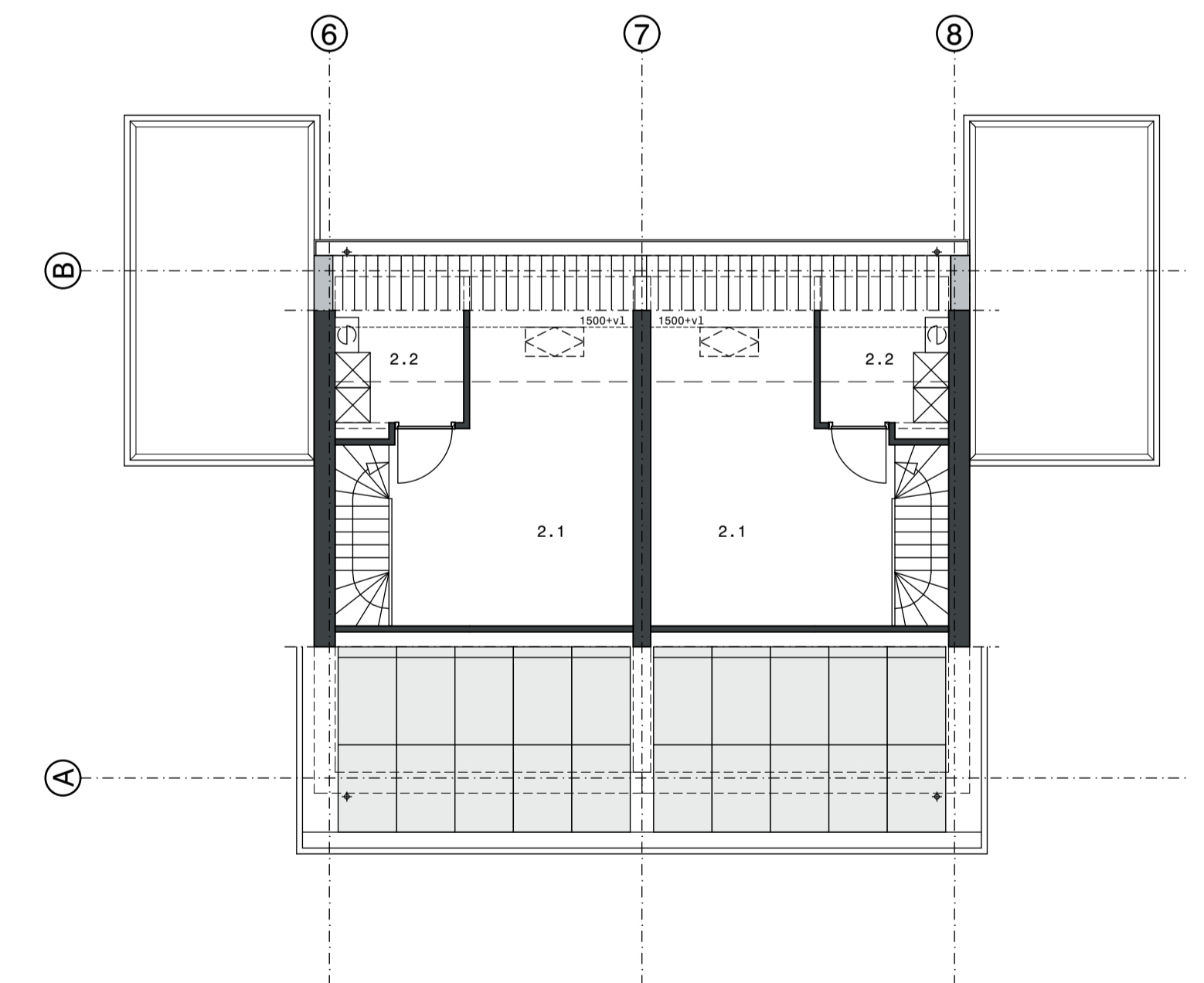
- Plattegrond 2e Verdieping -
